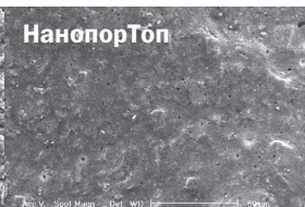
Обичайна мазилка
